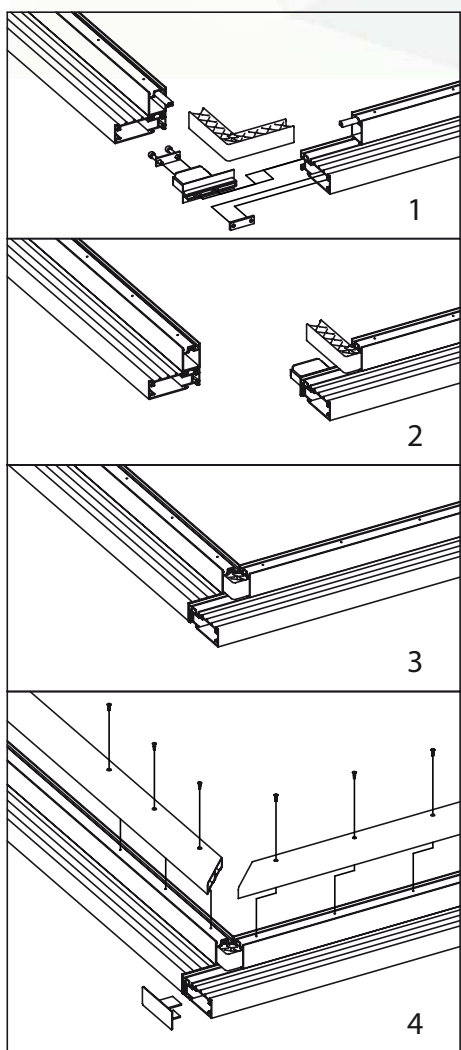
Schemat montażu
