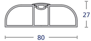
BU80+BUC80
